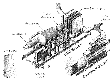
Фиг. 3 Ко-генератори (ORC) за утилизация на отпадъчната топлинна
